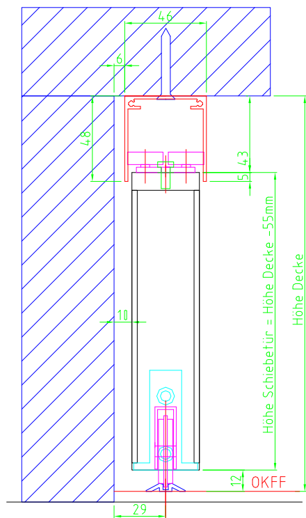
Bild 1 Deckenmontage
