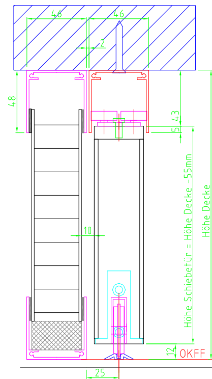
Bild 3 Montage mit Trennwand T38
