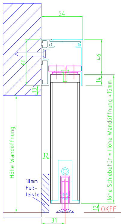
Bild 2 Wandmontage
